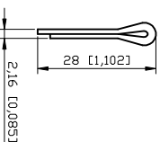
开口销 (Cotter key)
